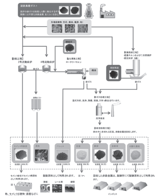
光和精鋳 廃棄物リサイクルフロー図
